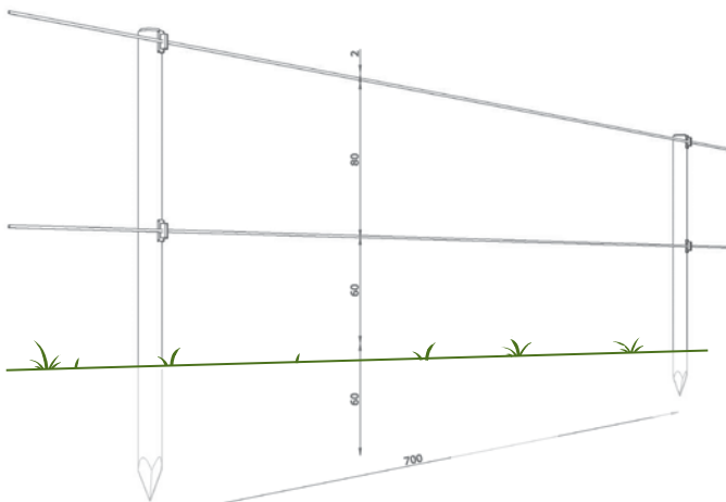
Hippolux-hegn med to tråde (Se Poda standard type C120)
