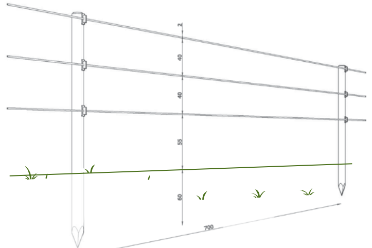
Hippolux-hegn med tre tråde (Se Poda standard type C140)
